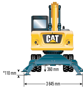
Podvozek s dvěma soupravami opěrných noh
