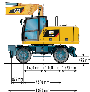
Podvozek s jednou soupravou opěrných noh a radlicí
