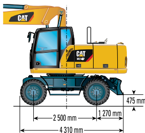
Podvozek pouze s radlicí
