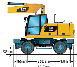
Podvozek s dvěma soupravami opěrných noh
