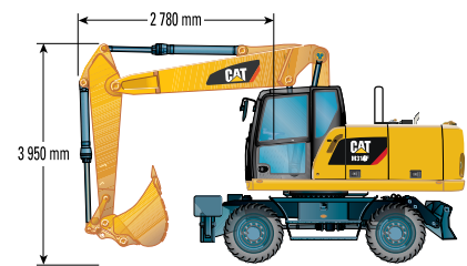
Poloha pro jízdu po komunikacích s násadou 2 300 mm
